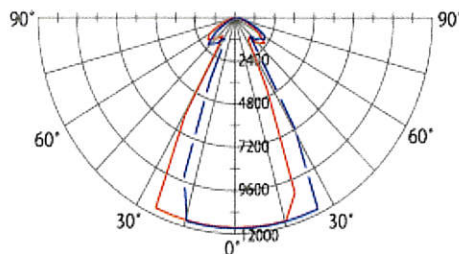
配光図・照度図(150W)
