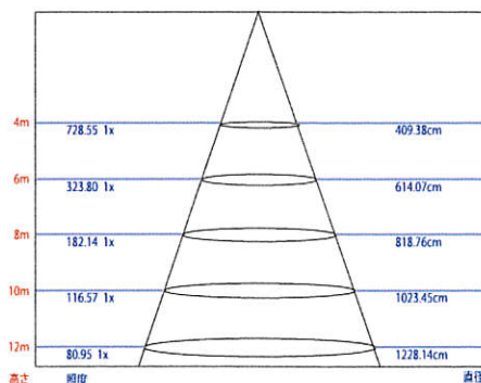
配光図・照度図(150W)
